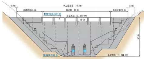
《玉来ダム下流断面図》
